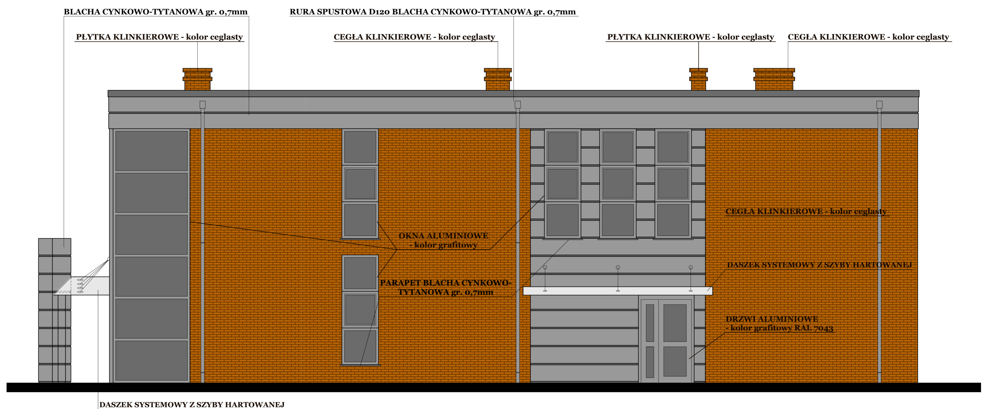
ELEWACJA POŁUDNIOWO-WSCHODNIA
